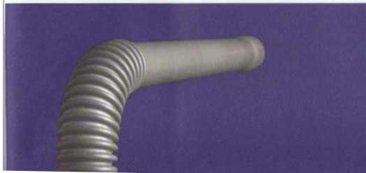
Flexydrain® PP-buis in combinatie met platte sifon voor douche (alle beelden doc. Plastiflex)
